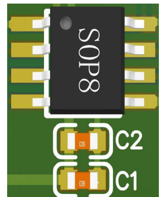
PCB 设计电容放置位
